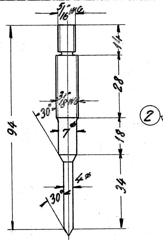
2 rensenål 10 \phi x 92 rustfrit st.
